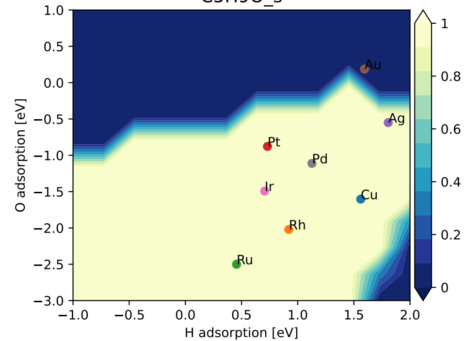
C5H9O_s
